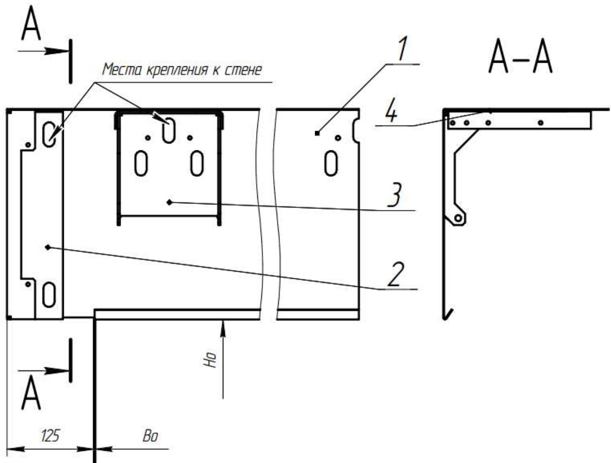
Рис 1. Схема монтажа первой секции короба: 1 – задняя угловая стенка, 2 – боковая крышка, 3 – кронштейн консоли, 4 – монтажная пластина. Обозначения: Bo – ширина проёма, Ho – высота проёма.
